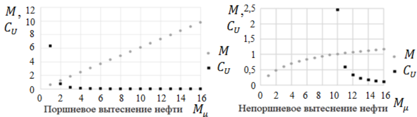
Рис. 10. Зависимость критериев устойчивости вытеснения нефти от отношения вязкостей для различных моделей вытеснения
