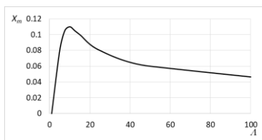
Рис. 16. Зависимость безразмерной глубины проникновения реагента в пласт от безразмерного коэффициента фильтрации
