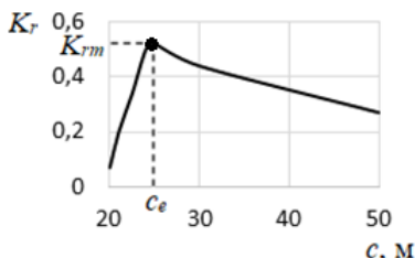
Рис. 9. Результаты определения эффективного расстояния между парами скважин для месторождения Fengcheng по критерию максимального коэффициента извлечения нефти
