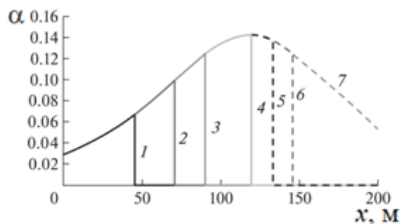
Рис. 20. Распределение концентрации частиц в трещине при D_f < 1 ( k = 1,6 \cdot 10^{-10} \text{ м}^2 ) в моменты времени 1,25 с (кривая 1), 2,5 с (кривая 2), 3,75 с (кривая 3), 6 с (кривая 4), 7 с (кривая 5), 8 с (кривая 6), 25 с (кривая 7) для модельного пласта
