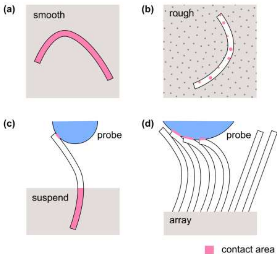
Рис. 1. Схематическое изображение некоторых конфигураций трибологических систем с гибкими одномерными наноструктурами: (a) контакт ННК с гладкой поверхностью (“smooth”), (b) контакт ННК с шероховатой поверхностью (“rough”), (c) частичный контакт свисающего (“suspend”) ННК с плоской поверхностью и зондом, (d) контакт упорядоченного наклоненного массива (“array”) ННК с зондом. Цветом обозначены участки непосредственного контакта тел (“contact area”).
