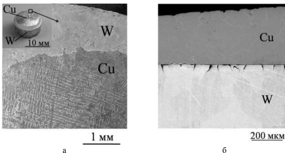
Рис. 1. Внешний вид образца Cu-на-W, полученного после плавления меди (а): на врезке выделена область поверхности образца, по стрелке показанная с большим увеличением; участок вертикального сечения образца (б)
