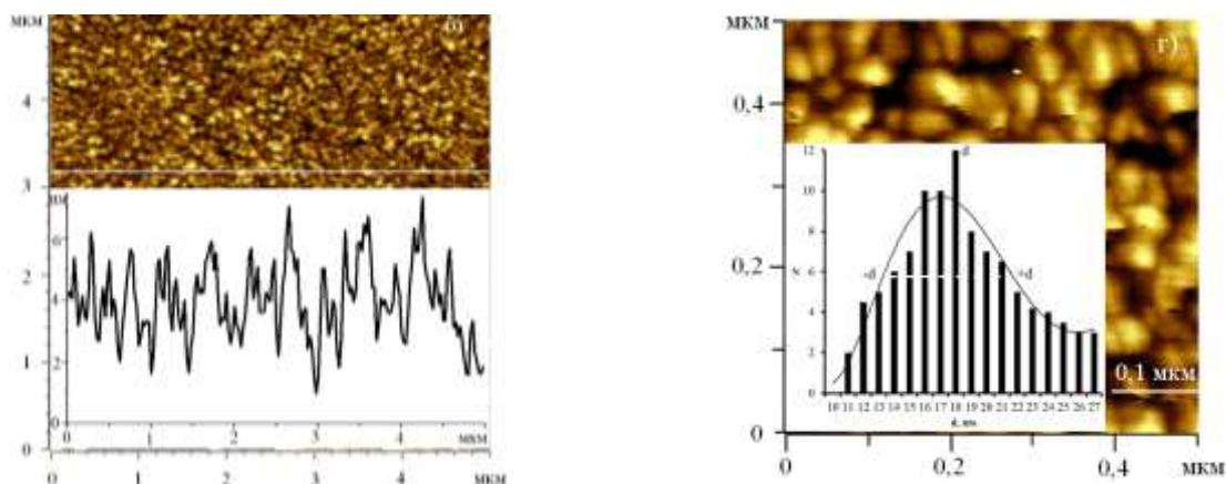
Рис. 3. АСМ изображения магнетронных нанопленок из \text{Bi}_2\text{Te}_3 : а) n -типа проводимости; б) p -типа проводимости с профилограммой; 0.5 \times 0.5 \text{ мкм}^2 с данными гранулометрического анализа в) n -типа проводимости; г) p -типа проводимости
