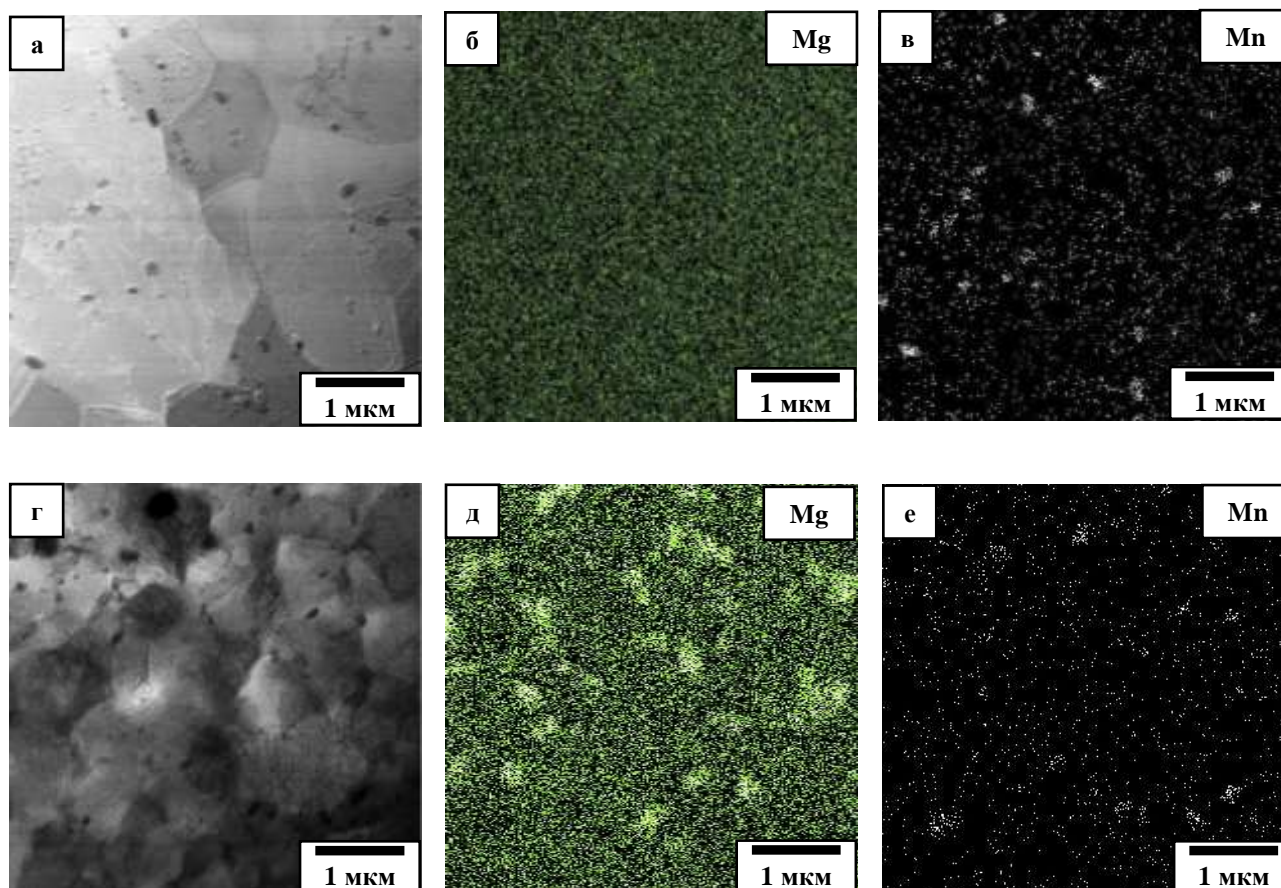
Рис. 1. Структура сплава 1570С, подвергнутого ВИК при 325°C (а-в); и 175°C (г-е) в состоянии после одноступенчатого отжига. Просвечивающая электронная микроскопия (а,г) и энергодисперсионный анализ (б,в,д,е)
