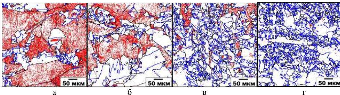
Рис.2. EBSD-карты границ зерен в криокатаном со степенью 30 (а), 50 (б), 70 (в) и 90% (г) никеле после получасового отжига при 400^\circ\text{C} . Красным цветом обозначены малоугловые границы, черным – высокоугловые, синим – двойниковые.
