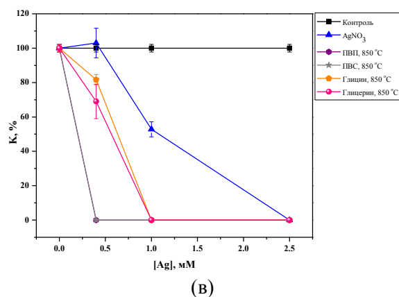
Рис. 1. Результаты исследования наноконпозиций \text{Al}_2\text{O}_3\text{-Ag} : (а) – СЭМ-изображение частиц серебра на поверхности агрегата оксида алюминия (ПВП, 850 °С); (б) – результаты РФА образца \text{Al}_2\text{O}_3\text{-Ag} , ПВП, 850 °С; (в) – результаты определения антибактериальной активности (в процентах роста колоний по отношению к контролю).
