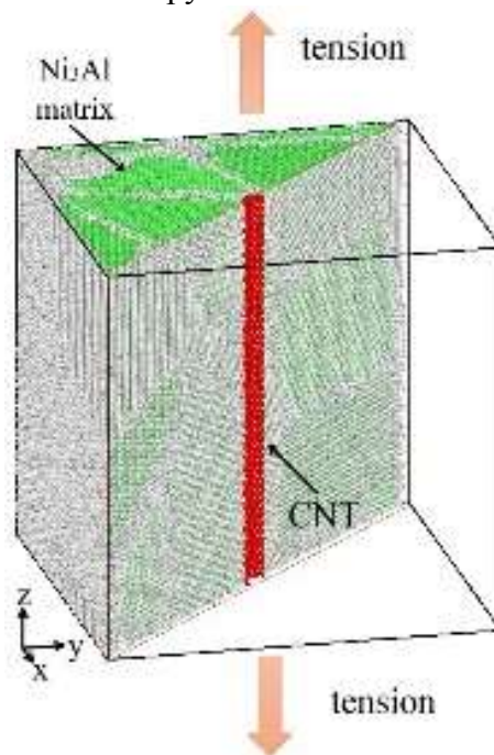
Рис. 1. Модель поликристалла Ni 3 Al с внедренной УНТ вдоль оси прикладываемой нагрузки
