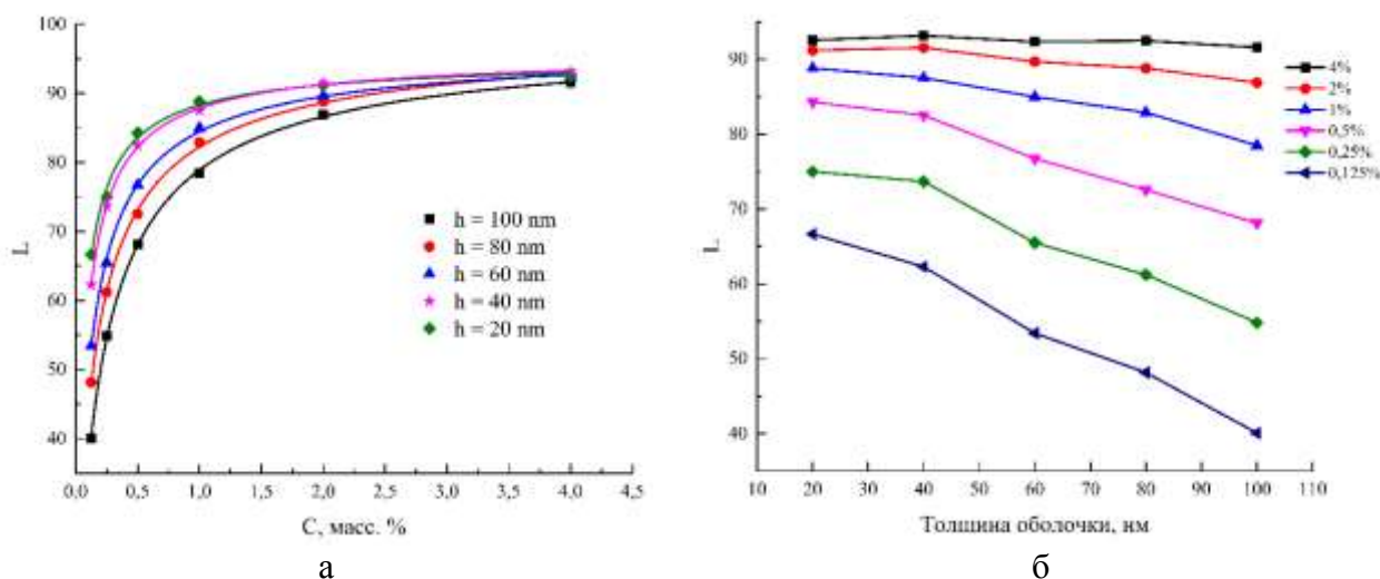
Рис. 2. Зависимости величины светлоты L суспензий полых частиц диоксида кремния в растворе глицерин-вода 1:1 от их массовой концентрации (а) и толщины оболочки (б).
