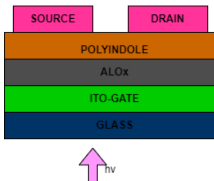
Рис. 1. Структура фототранзистора
