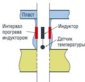
Рис. 1. Упрощённая схема проведения исследований с применением метода индукционного нагрева
