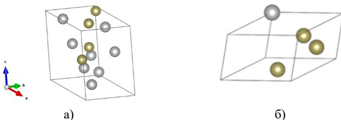
Рис. 1. Кристаллическая структура: (а) – Ag_8Te_4 , (б) – AgTe_3
