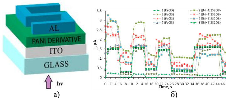
Рис. 1. а) Структура фоторезистора с плёнкой изучаемой производной анилина. б) Зависимость тока от времени облучения при напряжении 10 вольт и расстоянии от выхода излучения из оптоволоконного кабеля до образца 10 мм
