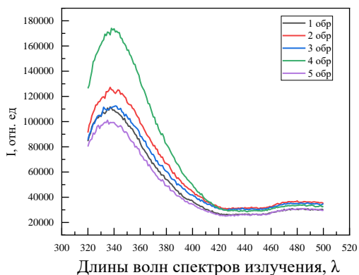
Рис. 2. Спектры возбуждения при \lambda возб. = 300 нм
