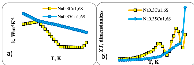
Рис. 1. Теплопроводность (а) и добротность ZT (б) образцов
