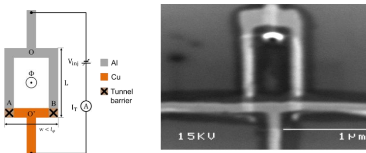
Рис. 1. Левая панель: схематическое представление интерферометра. Правая панель: микрофотография твердотельного интерферометра, полученная растровым электронным микроскопом
