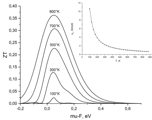
Рис. 2. Термоэлектрическая добротность и решеточная теплоемкость
