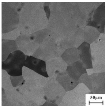
Рис. 1. Микроструктура сплава в литом состоянии
