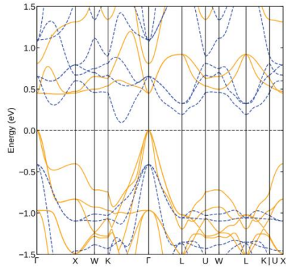
Рис. 1. Зонная структура FeVScSb
