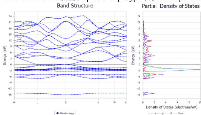
Рис. 2. Зонная структура \text{Cu}_2\text{Se} при температуре 673 К
