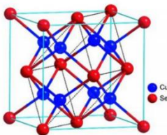
Рис. 1. ГЦК структура соединения \text{Cu}_2\text{Se}
