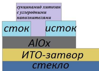
Рис. 1. Конструкция экспериментального полевого транзистора
