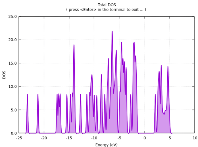
Рис. 2. График плотности состояний
