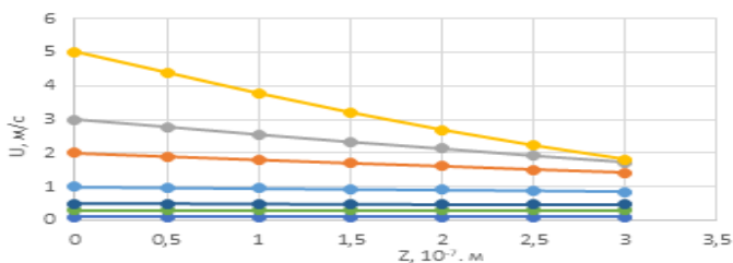
Рис. 1. Зависимость скорости молекул воды от расстояния от дрейфующего иона
