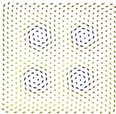
Рис. 1. Основное состояние пленки с четырьмя скирмионами
