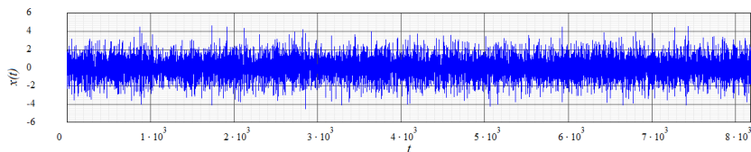
Рис. 2. Реализация синего шума с индексом СПМ, близким к 1
