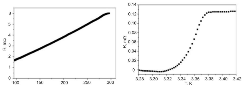
Рис. 1. Зависимости сопротивления от температуры R(T, I_{ac}=\text{const}) для тонкопленочной слоистой гетероструктуры In–PDP–In (а) в высокотемпературном диапазоне и (б) в области сверхпроводящего перехода. Измерения проводились в 4-х контактной конфигурации на переменном токе I_{ac}=1 мА на частоте 17 Гц методом фазочувствительного детектирования
