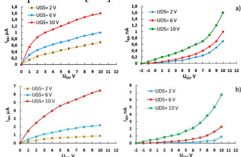
Рис. 1. Выходные и передаточные характеристики полевого транзистора с активным слоем: а) SCTS б) SCTS-GO
