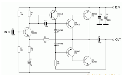
Рис. 1. Схема усилителя
