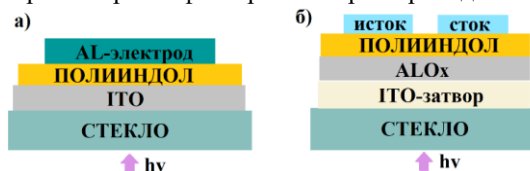
Рис. 1. Структура (а) фоторезистора и (б) фототранзистора
