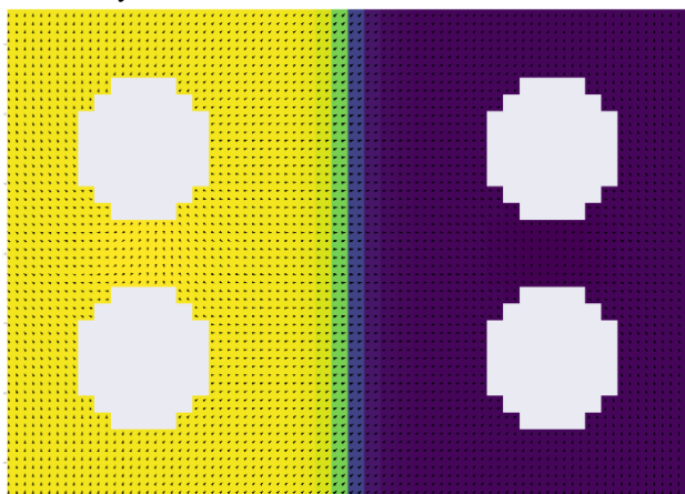
Рис. 1. Топологически защищенные структуры в плёнке с четырьмя отверстиями
