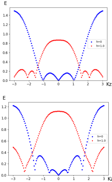
Рис. 1. Зависимость энергии от волнового вектора k_z со спиральной структурой по оси y в случае \theta = \frac{\pi}{3} , k_y = k_x = 0 , J_1 = 2 , J_2 = -1 , \langle S^z \rangle = 0.5 без внешнего магнитного поля h = 0 (синий цвет), с включенным магнитным полем h = 1 и g\mu_B = 1 (красный цвет). Слева: J_{mf} = 0.0 (модель однослойной магнитной пленки), справа: J_{mf} = 1.0 (модель системы, состоящей из магнитной и сегнетоэлектрической пленок)
