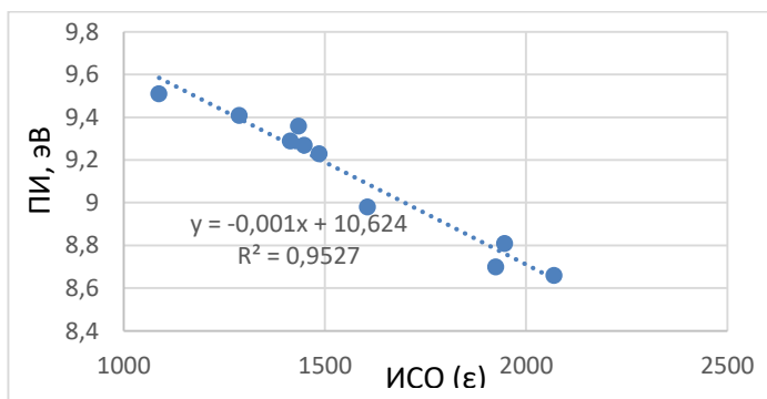
Рис. 1. Зависимость ИСО от ПИ органических красителей
