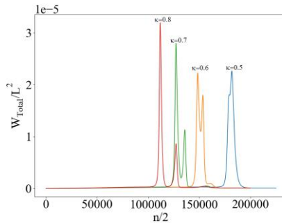
Рис. 1. Временное изменение общей диссипации
