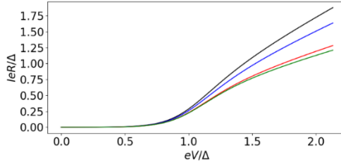
Рис. 2. Вольт-амперная характеристика NIS'S структуры.
