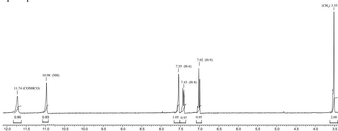
Рисунок 2.23. Спектр ЯМР 1 H 7-бром-1,5-дигидро-2H-хромено-[2,3-d]пиримидин-2,4(3H)-диона
