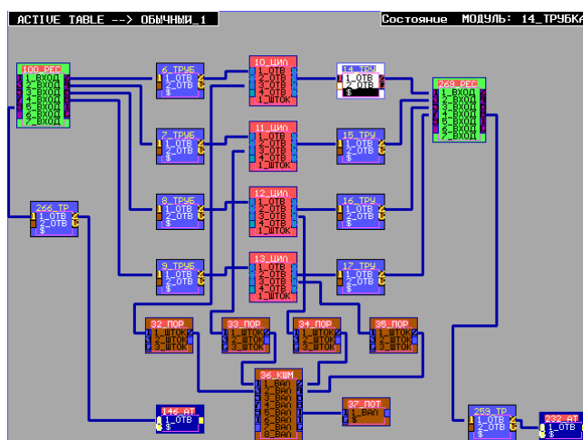
Рисунок 1.1 – Модель двигателя УЗАМ-1700 в СИМ «Альбея»
